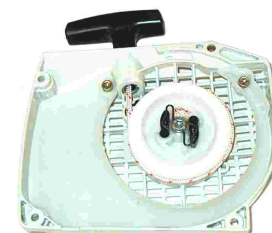
Art. 54.160.2368 Gruppo avviamento cpl adattabile a Starter cover (full) replaces Stihl 044 - 046
