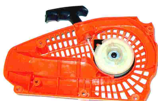
Art. 54.160.2370 Gruppo avviamento cpl adattabile a Starter cover (full) replaces Zenoah 2500
