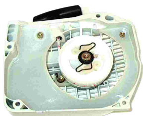
Art. 54.160.2369 Gruppo avviamento cpl adattabile a Starter cover (empty) replaces Stihl 066
