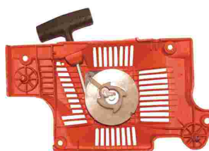
Art. 54.160.2352 Gruppo avviamento cpl adattabile Starter cover (full) replaces Husq. 51 - 55
