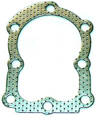
Art. 54.160.1670 Guarnizione testata cilindro adattabile a Cylinder-head gasket replaces Briggs & Stratton 2 + 3 HP orizzontali Rif. orig. (O.E.M.) 027167 • 27670
