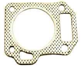
Art. 54.160.1681 Guarnizione testata cilindro adattabile a Cylinder-head gasket replaces Honda • GX 140 • Rif. orig. (O.E.M.) 12251-ZE1-800
