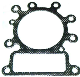
Art. 54.160.1676 Guarnizione testata cilindro adattabile a Cylinder-head gasket replaces Briggs & Stratton 13 • 14 • 15 HP • 15,5 INTEK -OHV verticali Rif. orig. (O.E.M.) 273280S
