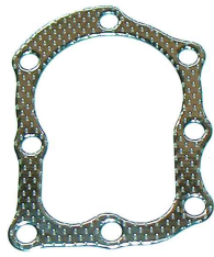
Art. 54.160.1671 Guarnizione testata cilindro adattabile a Cylinder-head gasket replaces Briggs & Stratton 3 + 3,5 HP verticali Rif. orig. (O.E.M.) 272170 • 272536
